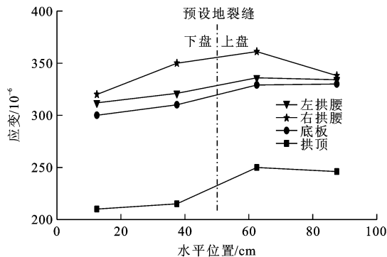
(a) 基于 El Centro 地震波的应变
