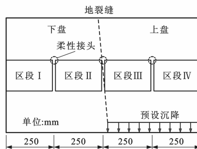
(b) 纵剖面
