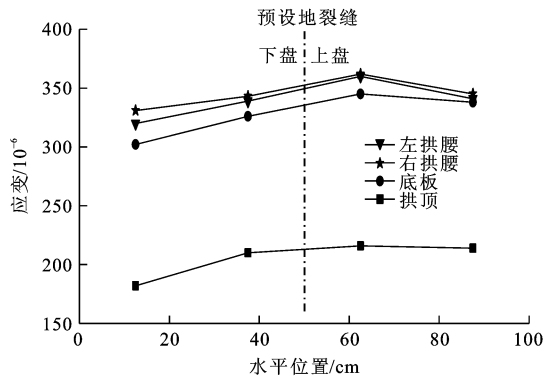
(b) 基于人工地震波的应变
