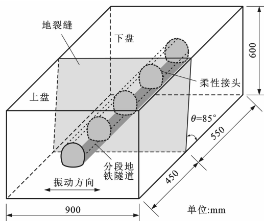
(a) 立体图
