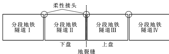
图2 分段柔性地铁隧道
